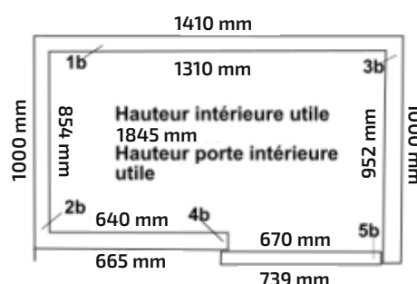
Vue de dessus intérieur cabine
